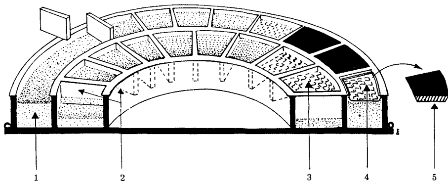
Schema van het granaat-cloisonné: 1. bevestigingsmiddel; 2. gouden celwand; 3. cloisonné cel; 4. goudfolie; 5. granaatsteen (uit: Arrhenius, 1985)
