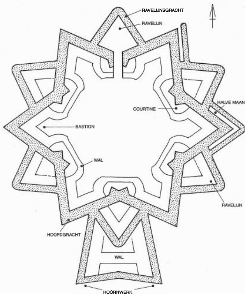
Reconstructietekening van de schans bij Bakkeveen
