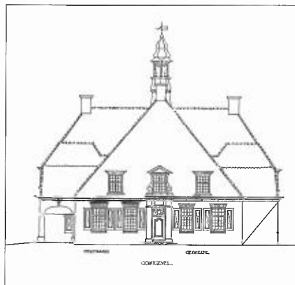
Diel ûntwerp-tekening ferbouwing 1922
